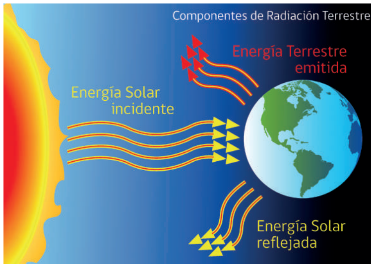
Esquema de balance radiativo entre el sol y la tierra
