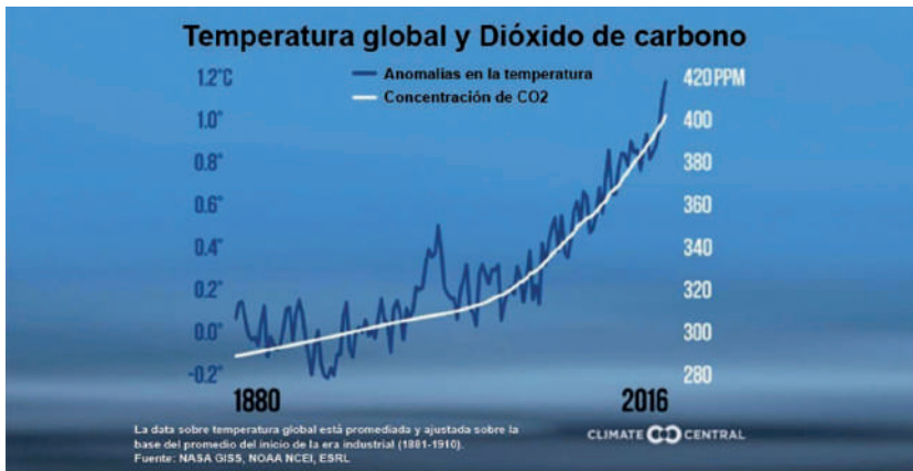
Aumento gradual de las temperaturas superficiales promedio en la tierra desde 1880
